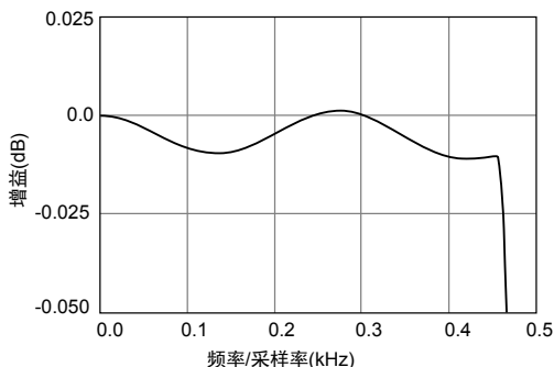
图 1. NI 9238 的典型通带响应
